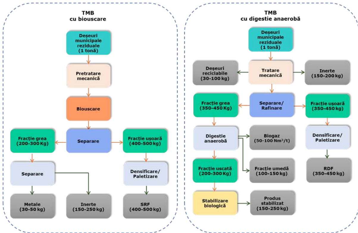
Figura 7-1: Fluxul tehnologic al instalațiilor TMB cu bioscarea și digestie anaerobă 51
